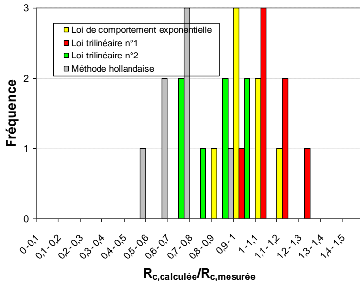
Figure 29. Distributions des ratios R_{c,calculé}/R_{c,mesurée} calculés à partir des trois lois de comportement et de la méthode hollandaise - Rouen
