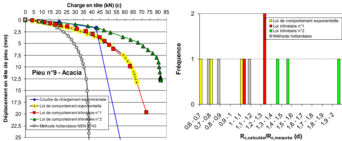
Figure 30. Comparaison des courbes de chargement expérimentales et théoriques des pieux n° 4 (a), n° 5 (b) et n° 9 (c) battus sur le plot expérimental de Cubzac-les-Ponts et distributions des ratios R_{c,calculée}/R_{c,mesurée} calculés à partir des trois lois de comportement et de la méthode hollandaise
