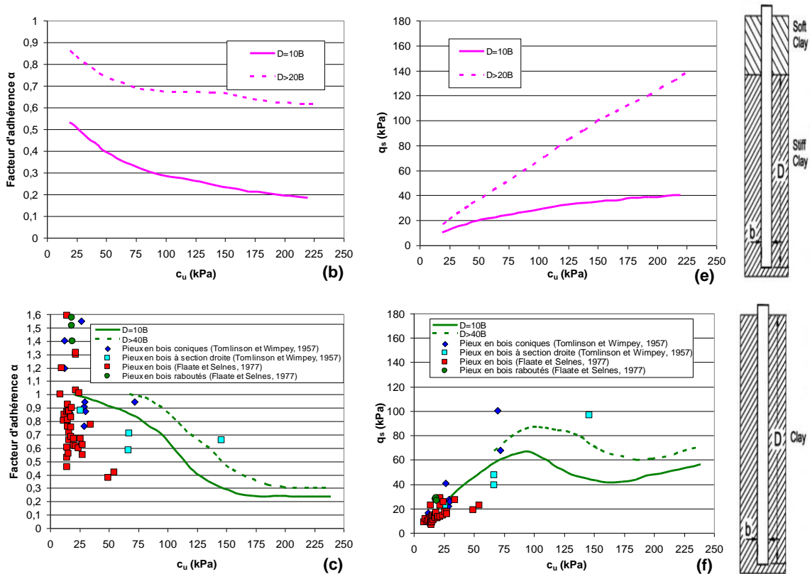
Figure 2. Évolution du facteur d'adhérence \alpha (a, b et c) et du frottement latéral unitaire (d, e et f) des pieux en bois en fonction de la résistance au cisaillement non drainée de l'argile (modifié d'après Tomlinson, 1994)
