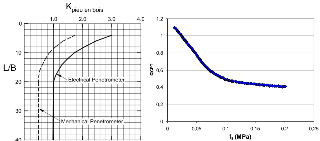
Figure 11. Évolution du facteur K en fonction du ratio L/B et du facteur \alpha' en fonction de f_s (modifié d'après AWPI, 2002 )
