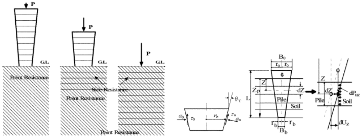
Figure 9. Discretisation du pieu en tranches rigides (Tominaga et Chen, 2006, cités par Tominaga et al., 2007)
