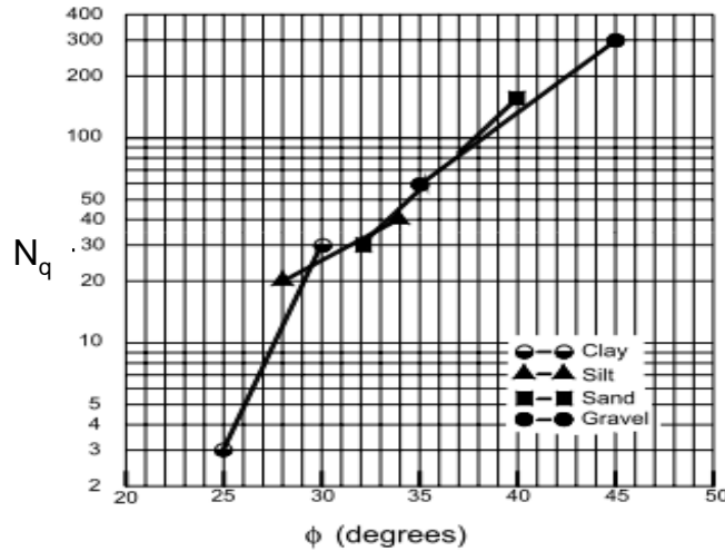
Figure 6. Estimation du facteur N_q en fonction de l’angle de frottement interne du sol (Fellenius, 1991)
