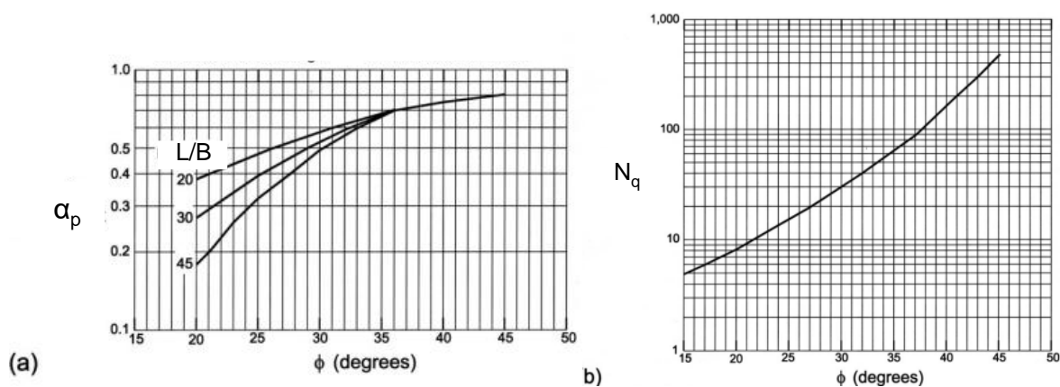
Figure 8. Évolution des facteurs \alpha_p (a) et N_q (b) en fonction de l’angle de frottement interne du sol (modifié d’après AWPI, 2002)
