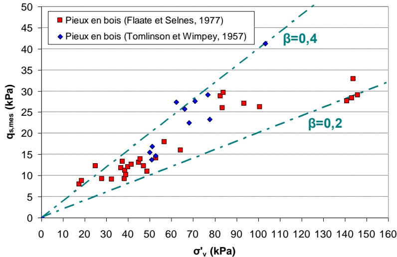
Figure 4. Plage de valeurs du facteur \beta (modifié d’après Flaate et Selnes, 1977)
