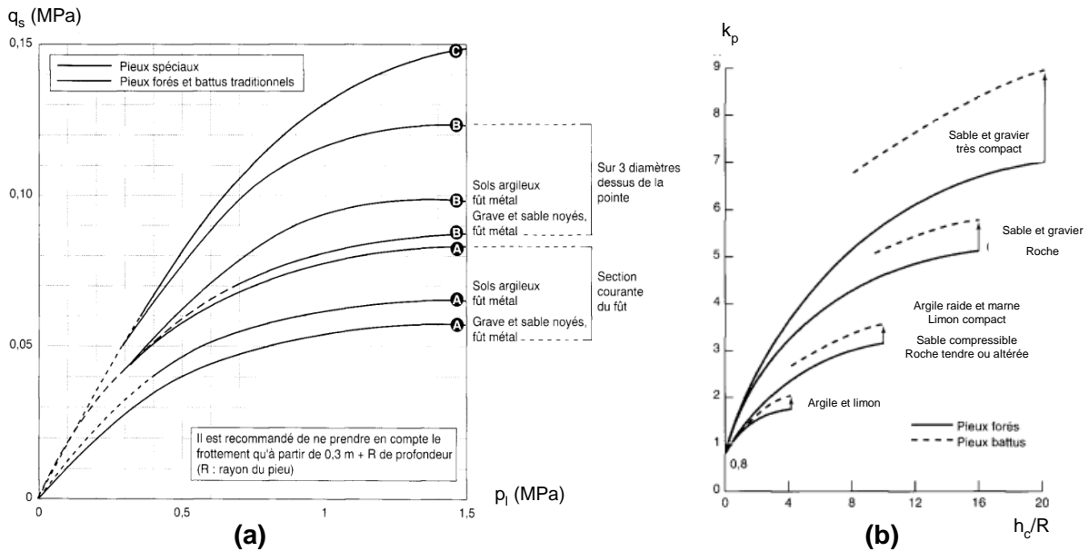
Figure 12. Evolutions de q_s en fonction de p_l (a) et de k_p en fonction de h_c/R (b) établies par Ménard, (1965) (modifié d'après Combarieu, 1996, 1999)
