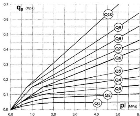
Figure 16. Evolution du frottement latéral unitaire limite q_s des pieux en fonction de la pression limite du terrain p_l ( Bustamante et Gianceselli, 2006 )
