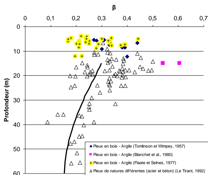
Figure 3. Évolution du facteur \beta en fonction de la profondeur (modifié d'après Le Tirant, 1992 )
