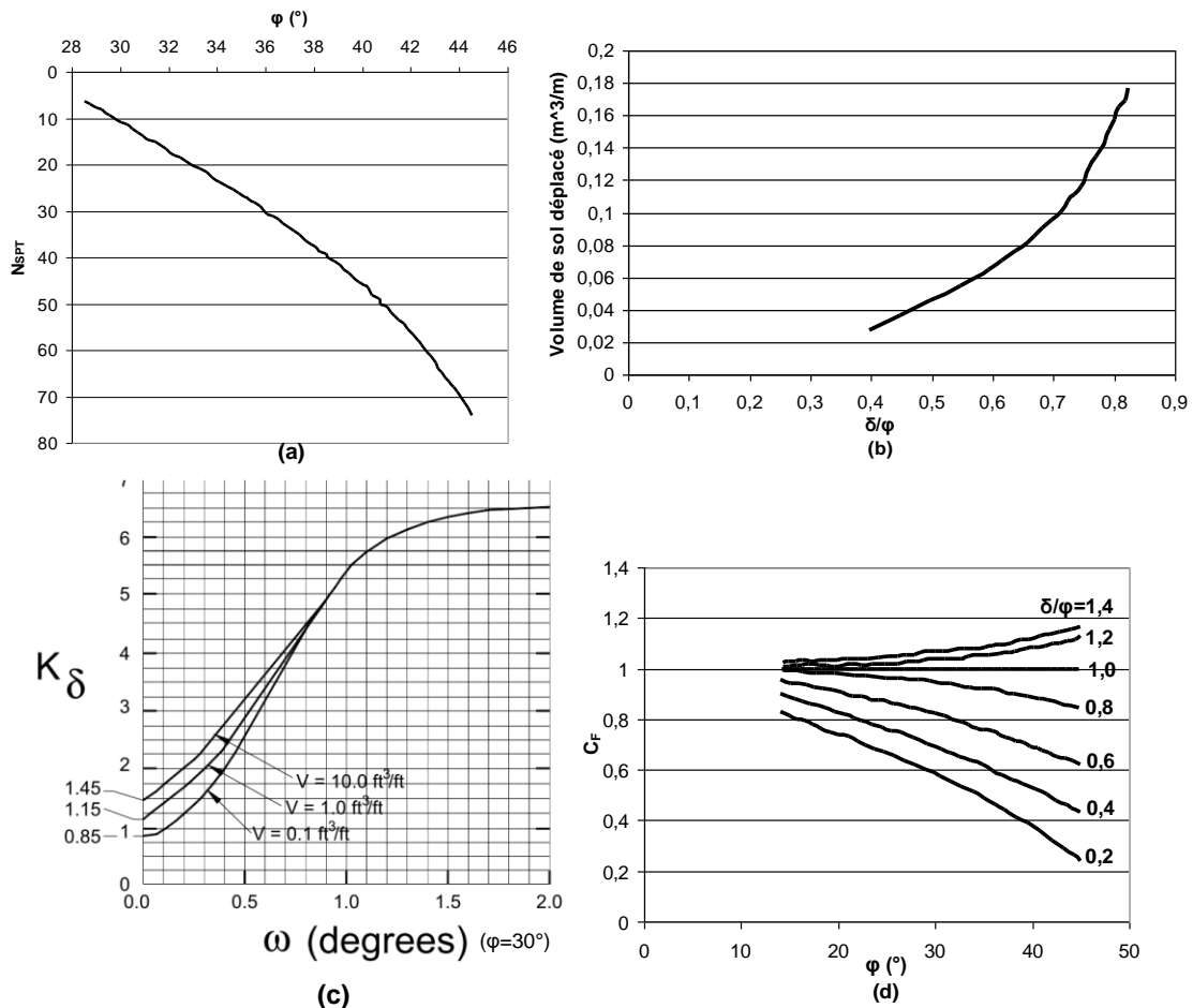
Figure 7. Évolution de l’angle de frottement du sol en fonction de N_{SPT} (a), du ratio \delta/\varphi en fonction du volume de sol déplacé (b), du facteur K_\delta en fonction du volume de sol déplacé et de la conicité des pieux (c), du facteur correcteur C_F en fonction de l’angle de frottement du sol (d) (modifié d’après AWPI, 2002)
