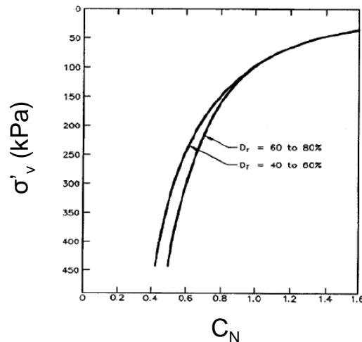
Figure 10. Évolution du facteur C_N en fonction de la contrainte verticale effective dans le sol (modifié d’après AWPI, 2002 )
